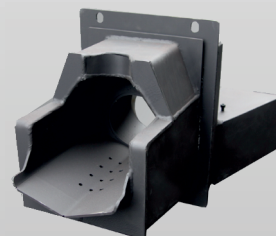
rynnové ohniště s zapalovačem
